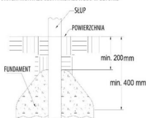
SYSTEM MONTAŻU SŁUPA METALOWEGO W BETONIE
