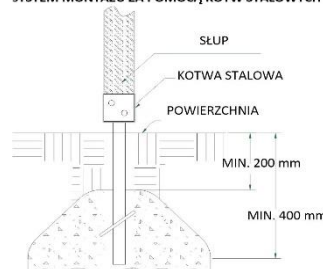
SYSTEM MONTAŻU ZA POMOCĄ KOTW STALOWYCH
