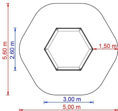
PIASKOWNICA | STREFA BEZPIECZEŃSTWA
