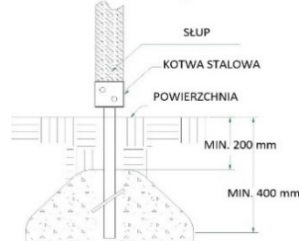
SYSTEM MONTAŻU ZA POMOCĄ KOTWY STAŁOWYCH
